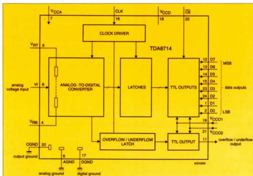
Blokdiagram van de TDA 8714.
