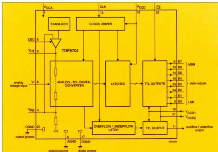
Blokdiagram van de TDF 8704.
